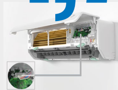
Abrir el cuadro eléctrico y desconectar los motores del ventilador, de las lamas y del ionizador
